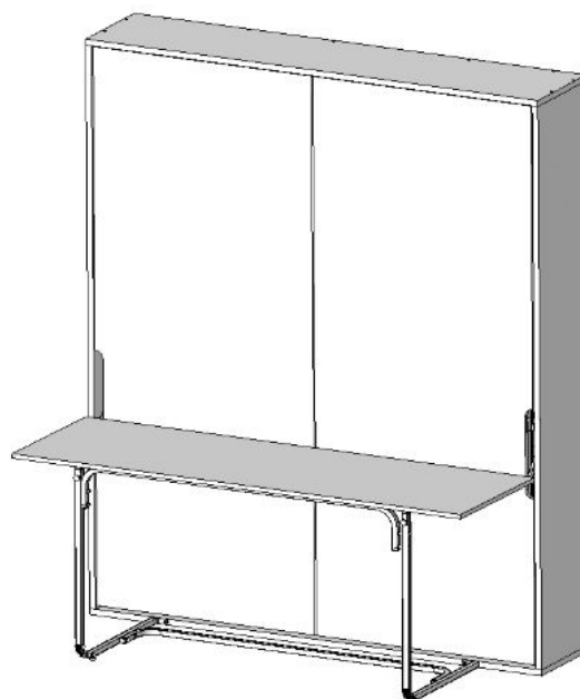
Рис.21.2 Стол разложен
