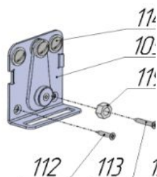
Рис.10.1 Закрепление при установке механизма на ЛЕВОМ щите короба
