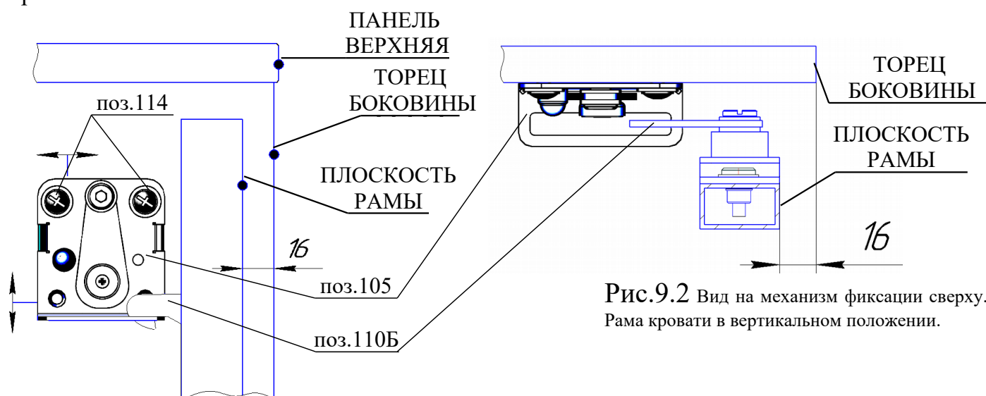
Рис.9.1 Вид на механизм фиксации изнутри короба. Рама кровати в вертикальном положении.
