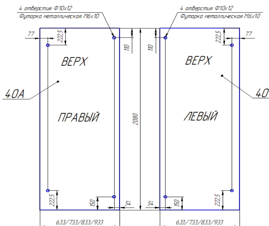
Рис.29 Места установки футорок на щитах декоративных
